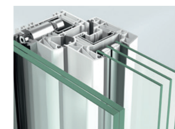
Befestigung mittels Hohlkammer-Dübel (bei geöffnetem Fenster unsichtbar)
