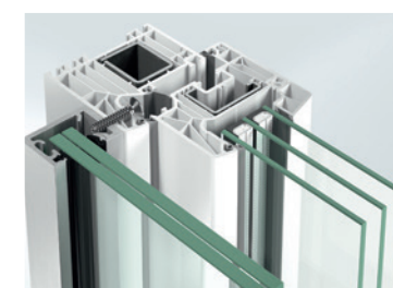
Befestigung mittels Falzleiste (bei geöffnetem Fenster sichtbar)
